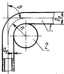
Загиб отрезков труб
